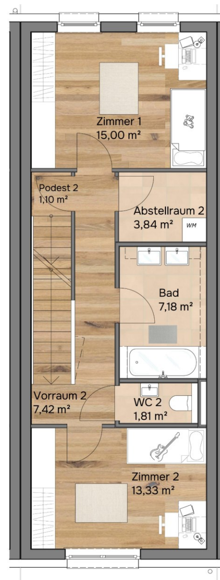
1.Obergeschoss Raumhöhe 2,53 m
